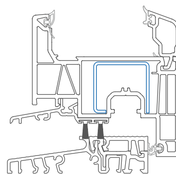
Elegantný prah balkónových dverí so šikmou zasklievacou lištou · Obr. 1 : 2
